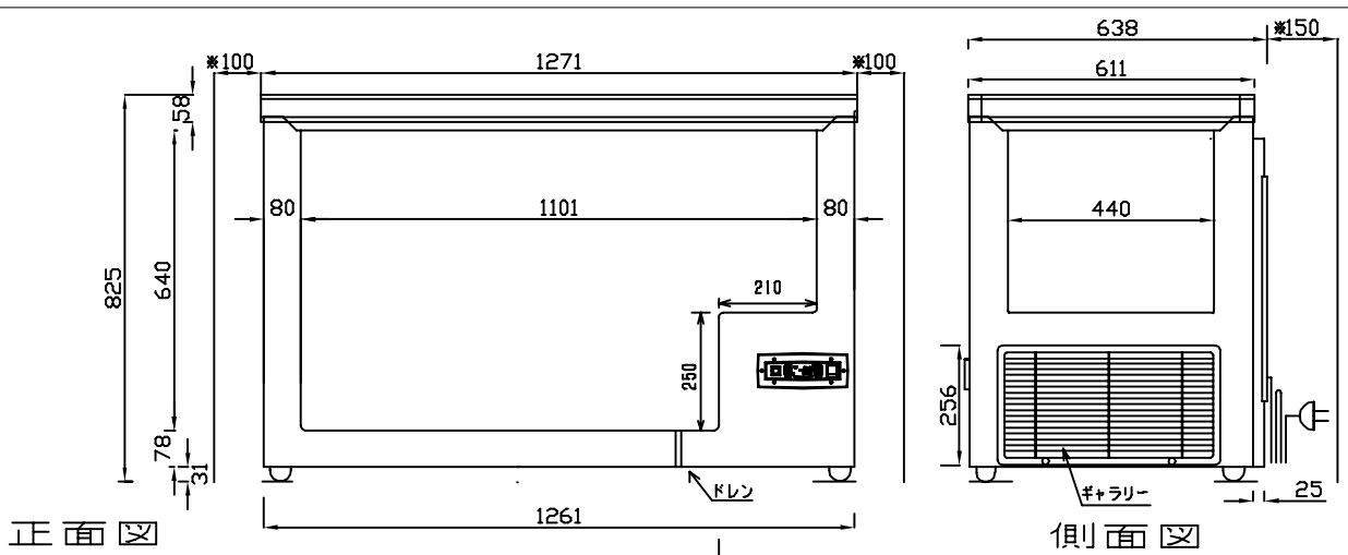
ドレン位置 上から見て 正面 手前
