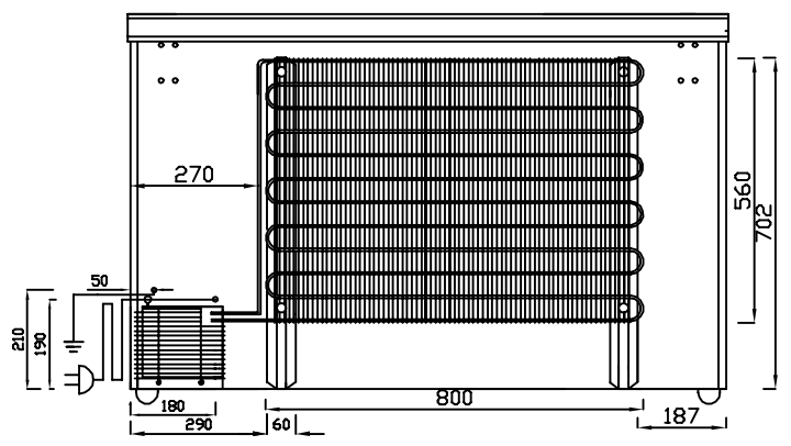
背面図
