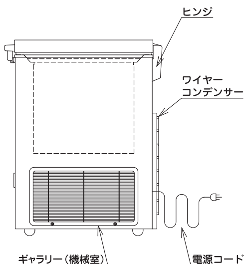
右側面図
